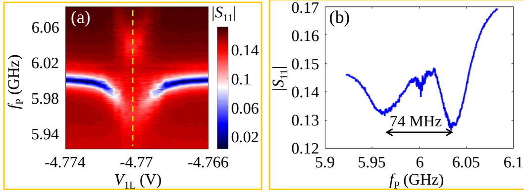
图 3.13 (a) DQD1 的量子点隧穿速率 2t_c/\hbar 接近腔频 \omega_r 时的真空 Rabi 劈裂。(b) 在失谐量为 0 处扫描的频谱, 可以提取得到耦合强度 2g_0/2\pi = 74 \text{ MHz} 。
