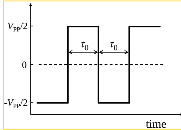
图 4.3 方波脉冲及其参数。
