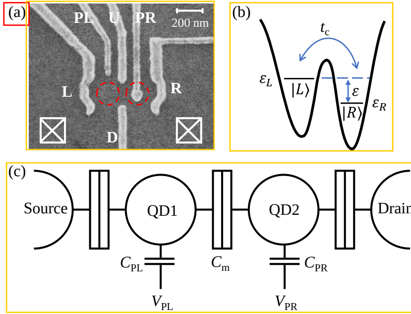
图 2.4 (a) 量子点金属电极电镜图。通过给电极 L、PL、U、PR、R 和 D 施加合适的偏置电压，会在两个虚线圆圈所指示的位置处形成量子点。(b) 双量子点束缚势示意图。电荷态 |L\rangle 和 |R\rangle 之间以隧穿速率 t_c 耦合，两点之间的电势差为失谐量， \varepsilon_L - \varepsilon_R = \varepsilon 。(c) 双量子点电路示意图。两点之间通过电容相互耦合，并各自耦合到相邻的源漏上。通过电极 PL 和 PR 和可以调节两个点内的电势。
