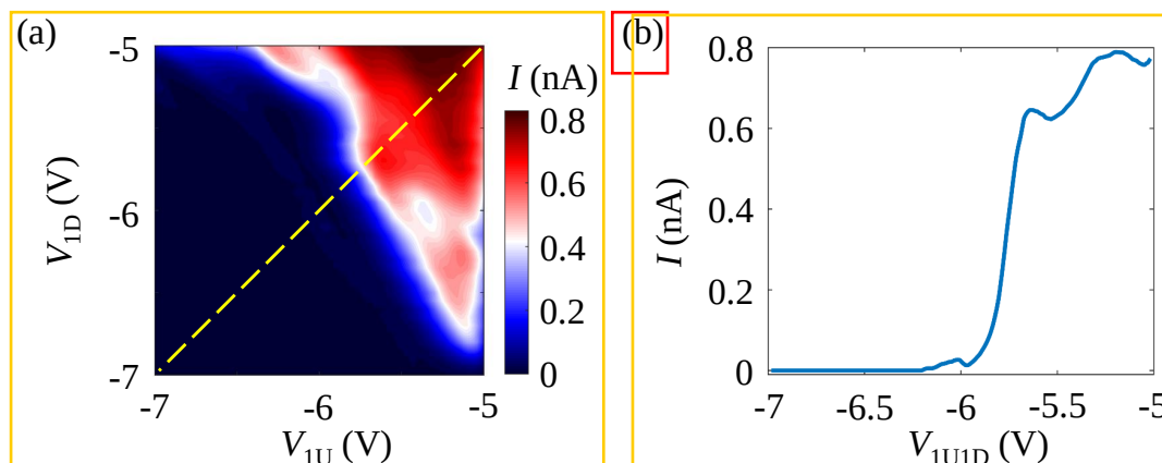
图 3.8 DQD1 的电极 U 和电极 D 之间的输运截止电压。(a) 扫描输运电流 I 随这两个电极电压变化的相图。(b) 沿相图的斜对角拉线得到电流-电压关系图，用来确定截止电压大小。
