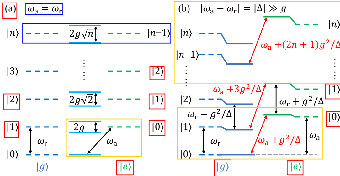
图 2.2 Jaynes-Cummings 哈密顿量的能级示意图。虚线是未耦合系统的本征能量, 左侧虚线对应比特处于基态 |g\rangle , 右侧对应比特处于激发态 |e\rangle , |n\rangle 为光子数态。实线是比特与腔光子在电偶极相互作用下的能级。(a) 比特与谐振腔共振, \omega_a = \omega_r 时, 能级劈裂形成新的本征态, 劈裂大小正比于 2g\sqrt{n} 。(b) 在色散极限区, |\omega_a - \omega_r| \gg g , 腔频受到比特影响发生偏移, \omega_r' \approx \omega_r \pm g^2/\Delta 。而原子的有效频率为 \omega_a' \approx \omega_a + (2n+1)g^2/\Delta 。
