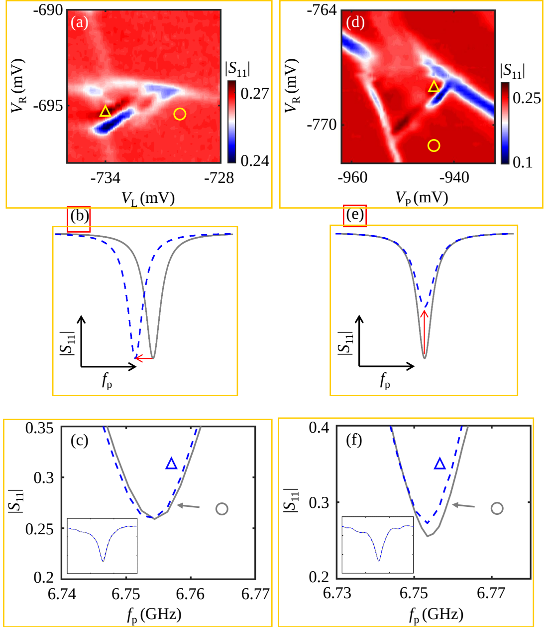
图 5.4 (a),(d) V_{SD} = 0.5 \text{ mV} 时测量腔幅值信号得到的电荷稳定图，用三角形标记出了增益区域，用圆形标记出了库伦阻塞区。(b),(e) 腔频偏移与量子点发光导致的腔信号幅值增益示意图。(c),(f) 在增益区域（虚线）和库伦阻塞区（实线）测量得到的频谱信号，放大展示了谐振谷附近的细节。左下角插图为完整的频谱曲线，几乎重叠在了一起。
