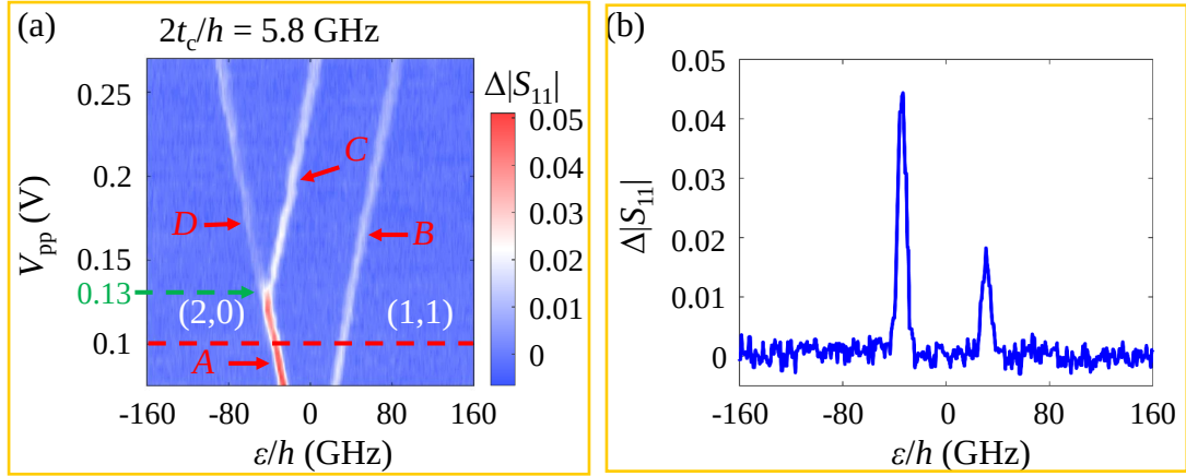
图 4.4 (a) 反射幅值信号 \Delta|S_{11}| 随失谐量 \epsilon 和脉冲电压 V_{pp} 变化的激发谱，数据已经经过处理扣除了库伦阻塞区的本底。(b) 沿幅值谱图中 V_{pp} = 0.1 \text{ V} 的水平截线。
