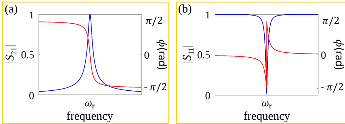
图 2.9 透射式 (a) 和反射式 (b) 谐振腔的幅值谱与相位谱示意图。
