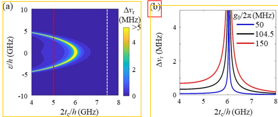
图 4.7 (a) 频率偏移 \Delta v_r 随 2t_c 和 \epsilon 变化的模拟图。左侧虚线和右侧虚线分别对应图 4.6(a) 和 (b) 激发谱的隧穿耦合速率 2t_c 。其它参数和实验一致。(b) 沿 (a) 图中零失谐量耦合强度 g_0/2\pi = 50 MHz (下方蓝色曲线)、 g_0/2\pi = 104.5 MHz (中间黑色曲线) 和 g_0/2\pi = 150 MHz (上方红色曲线) 时的 \Delta v_r - 2t_c 关系曲线。
