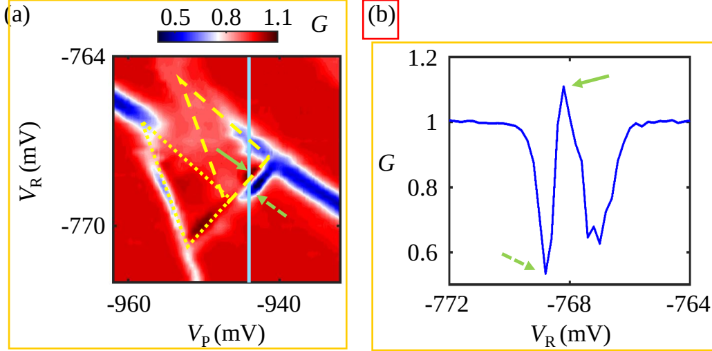
图 5.3 (a) 源漏偏置 V_{SD} = 0.5 \text{ mV} 时, 以电极电压 V_P 和 V_R 为扫描参数, 测量腔信号增益 G 得到的稳态图。其中上侧的偏压三角形轮廓由虚线标出, 下侧的偏压三角形轮廓由点线标出。实线箭头所指的区域腔信号幅值增强, G > 1 ; 虚线箭头所指的区域腔信号幅值被抑制, G < 1 。(b) 沿图 (a) 中 V_P = -944 \text{ mV} 截取的一条竖线。尖峰处对应光子发射, 而左侧低谷对应光子吸收。
