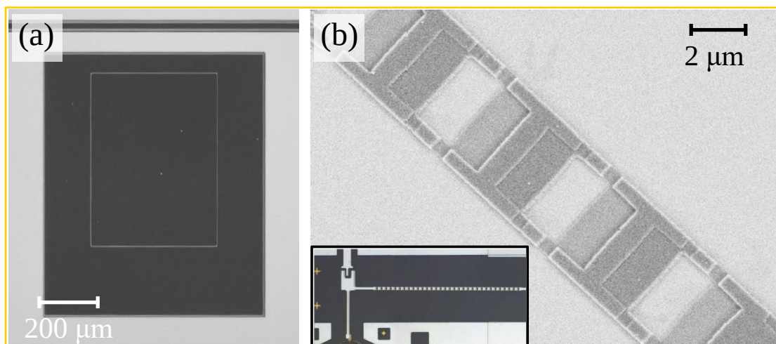
图 1.2 高阻抗超导谐振腔的扫描电子显微镜图。(a) 由 8 nm 厚的 NbTiN 薄膜制备而成的纳米线腔，线宽为 100 nm，围成了矩形形状。白色为 NbTiN 薄膜，黑色对应薄膜被刻蚀掉之后的衬底颜色。图片引自 [61]。(b) 超导量子干涉器件阵列构成的微波腔。左下角插图是量子点与腔耦合的整体结构图。图片引自 [51]。
