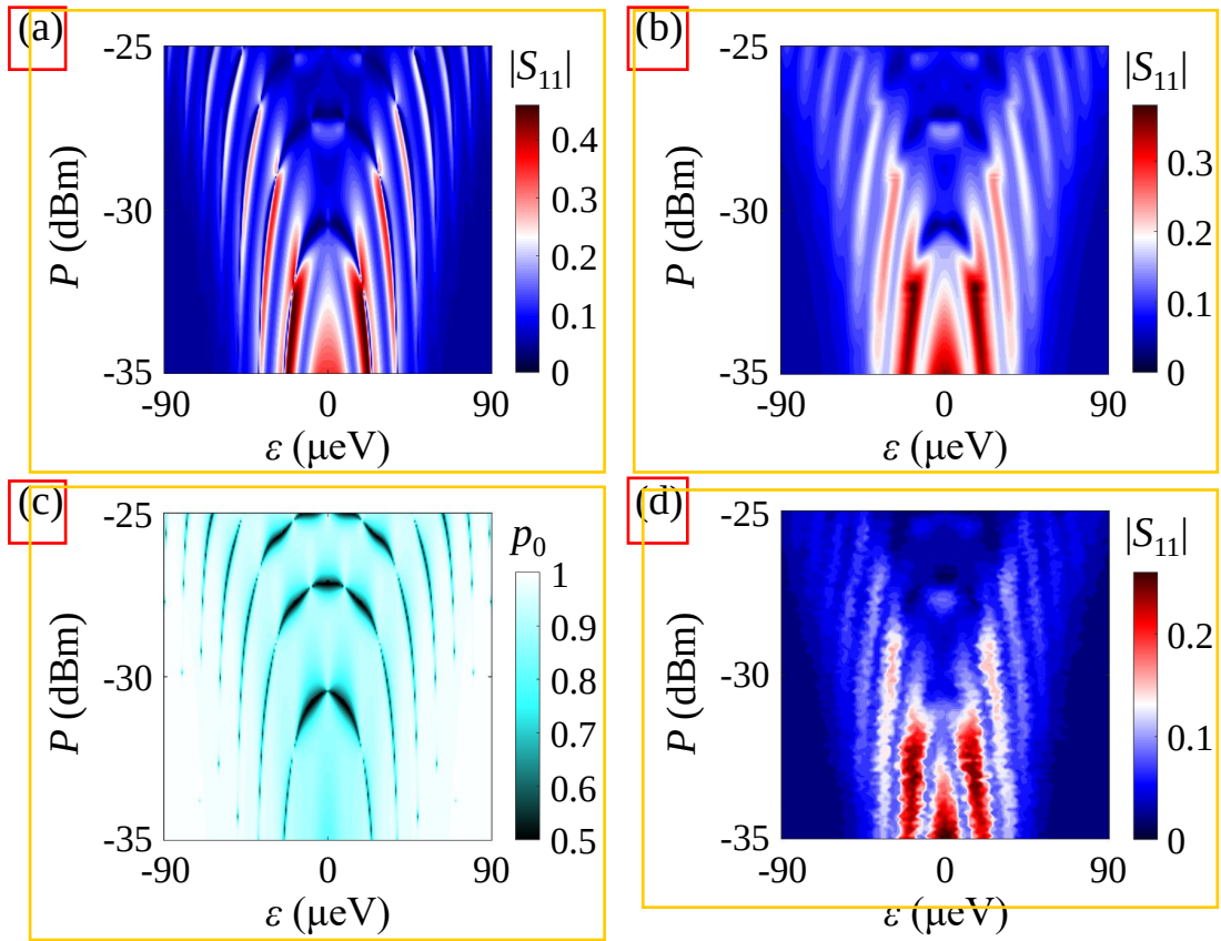
图 6.7 (a) 驱动频率 f_d = 2.27 \text{ GHz} 在接近三分之一谐振频率处的理论预言结果，驱动功率 P = -29 \text{ dBm} ，对应幅值 A_d = 45 \text{ } \mu\text{eV} 。(b) 相同的数值计算，但是额外考虑了失谐量 \varepsilon 具有 2.5 \text{ } \mu\text{eV} 的噪声展宽。(c) 理论计算的 Floquet 态 |\phi_0\rangle 平均布居。(d) 驱动频率 f_d = 2.27 \text{ GHz} 时的谐振腔响应实验结果。
