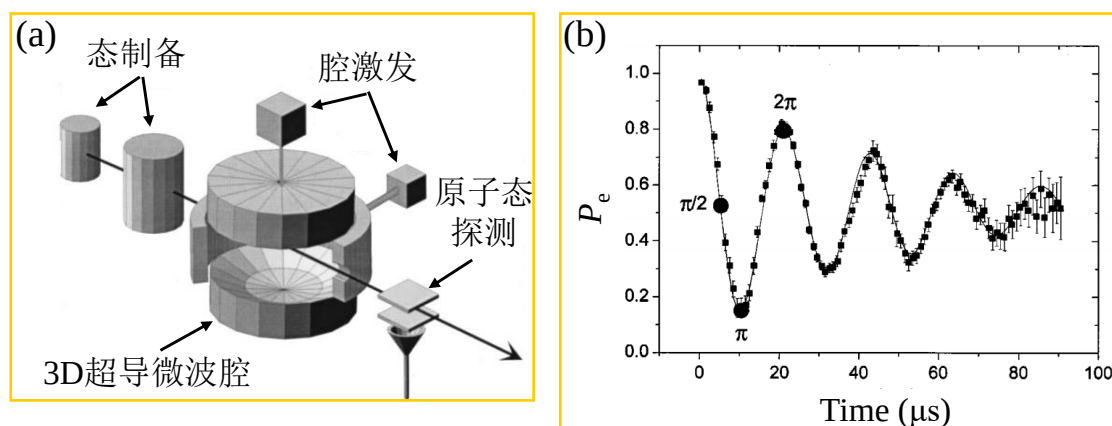
图 1.1 腔量子电动力学的 Rydberg 原子实验。(a) 样品装置图。原子在左侧被初始化到激发态上, 然后经过一个 3D 微波谐振器并被冷却到 \sim 1\text{ K} , 与腔内的光子相互作用, 穿过谐振腔后被右侧的测量装置探测到。(b) 在 Rydberg 原子系统中首次观测到的真空 Rabi 振荡。 P_e 表示原子处于激发态的概率。图片引自文献 [5]。
