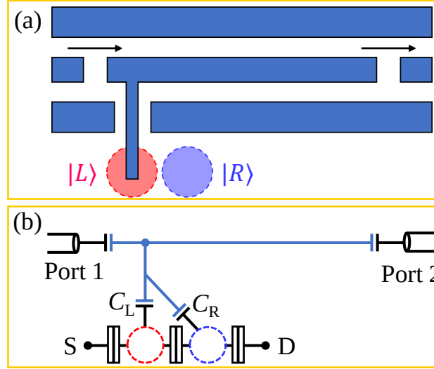
图 2.13 微波谐振腔与双量子点的耦合。(a) 耦合结构示意图。(b) 耦合电路示意图。
