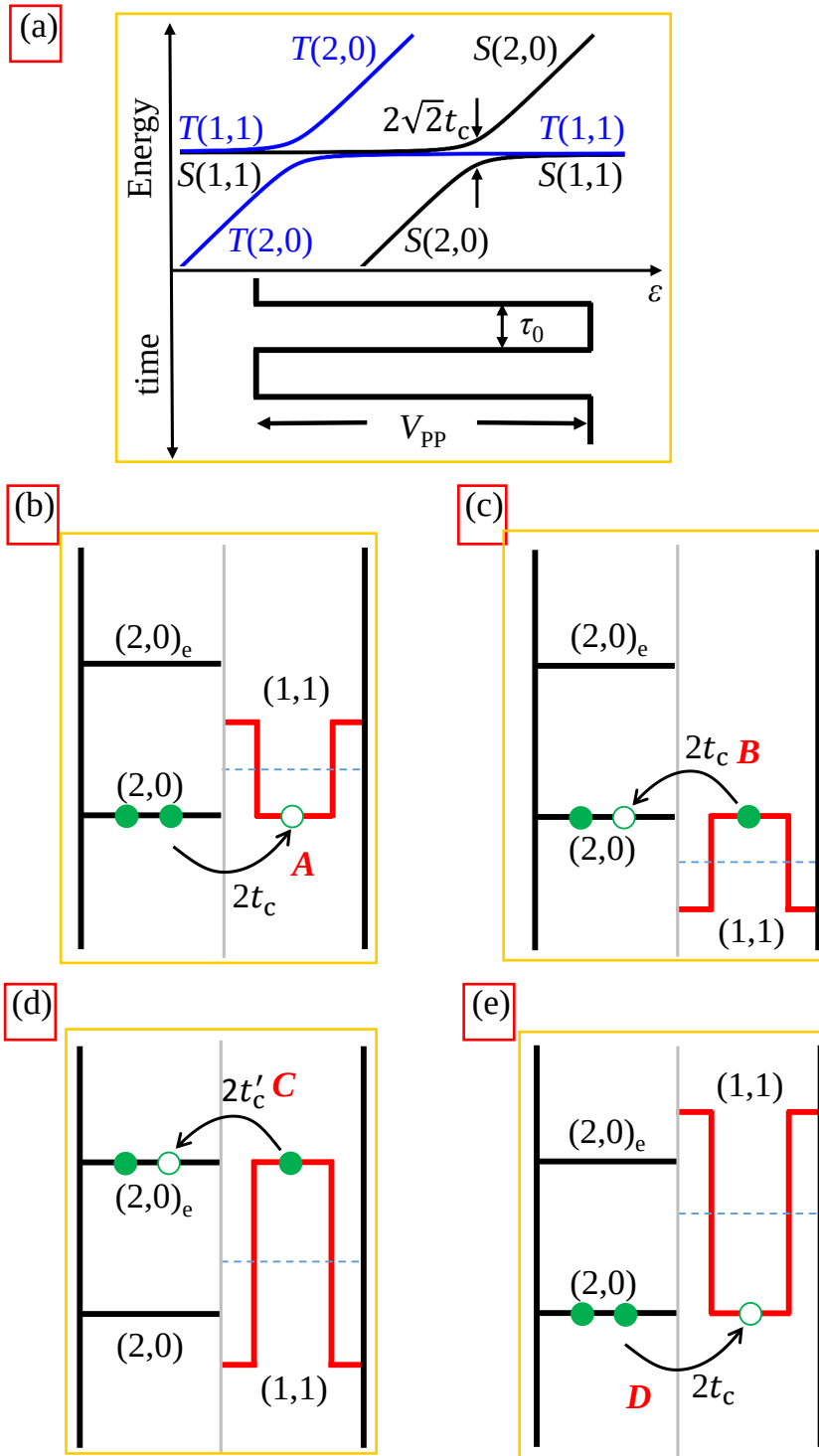
图 4.5 给双量子点施加方波脉冲后，电子的能级跃迁示意图。(a) 上侧：无外加磁场时的双电子自旋态的能级示意图。下侧：方波脉冲引起失谐量 \epsilon 随时间变化的示意图。(b)–(e) 在图4.4(a) 中跃迁线 A、B、C 和 D 对应的能级跃迁示意图。
