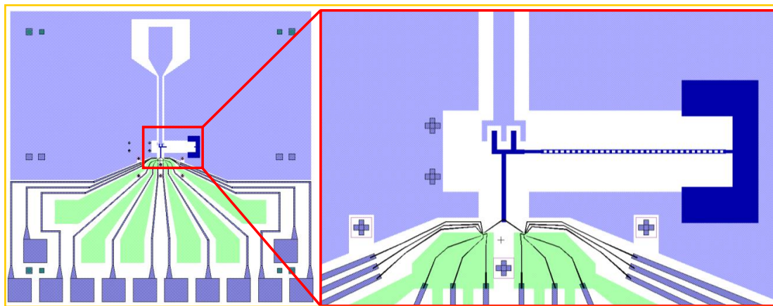
图 3.1 SQUID 阵列谐振腔和 GaAs 两个双量子点耦合结构的设计图。
