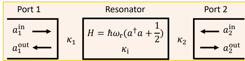
图 2.8 共面波导传输线谐振腔的二端口网络示意图。
