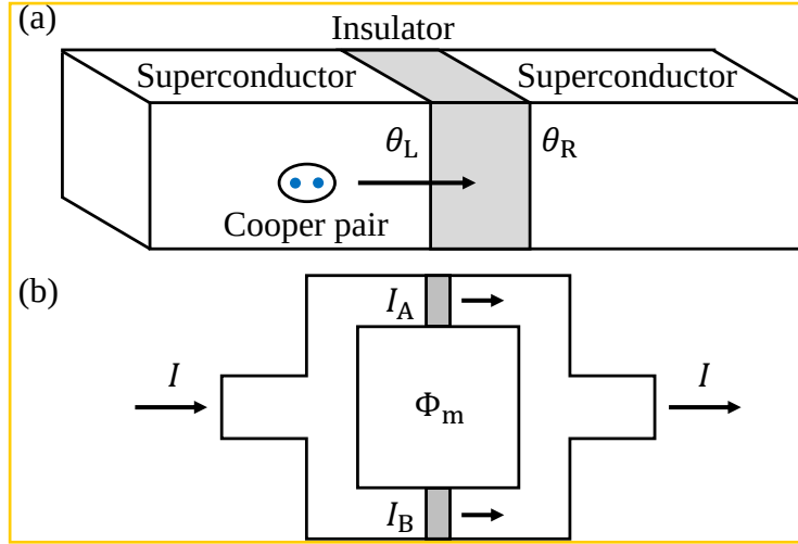
图 2.11 (a) 约瑟夫森结结构示意图。(b) SQUID 结构示意图。由两个约瑟夫森结并联组成。
