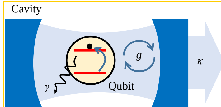
图 2.1 腔量子电动力学系统示意图。原子与腔内光子相互作用速率为 g ，光子的耗散速率为 \kappa ，比特的退相干速率为 \gamma 。
