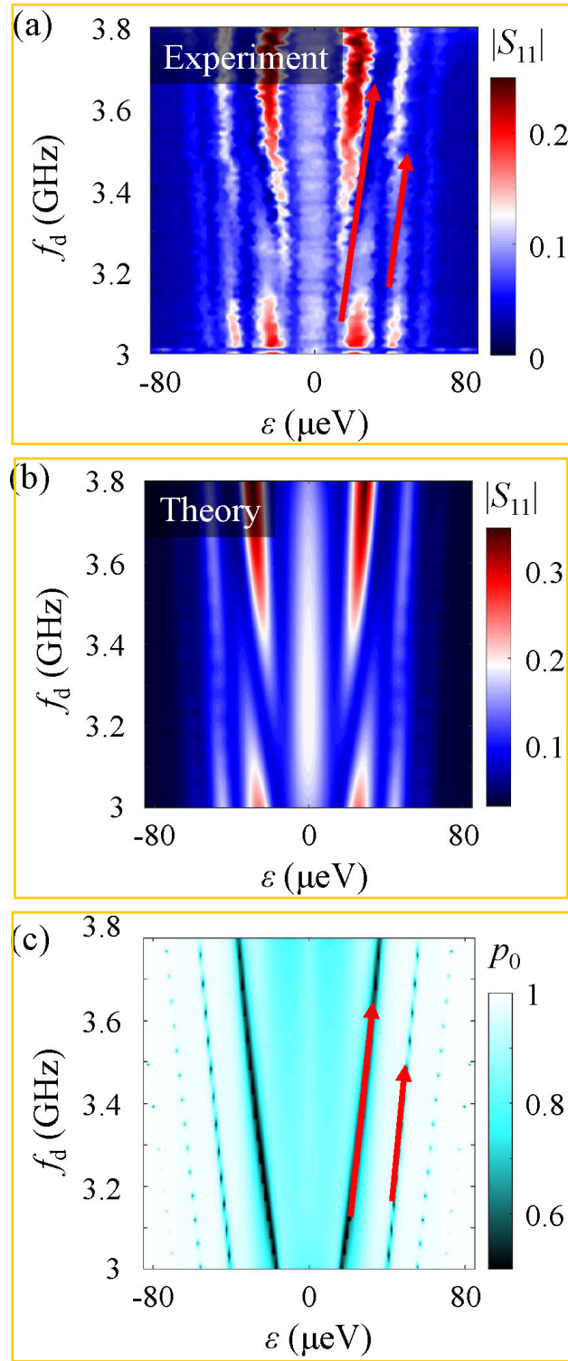
图 6.4 (a) 谐振腔反射信号 |S_{11}| 以失谐量 \varepsilon 和驱动频率 f_d 为函数扫描的 LZSM 干涉谱, 驱动功率 P = -36 \text{ dBm} , 2t_c/h = 6.2 \text{ GHz} 。红色箭头指出了“月牙”的演化方向。(b) 数值模拟结果, 模拟参数与 (a) 中的实验参数相同。(c) 理论计算的 Floquet 态 |\phi_0\rangle 的平均布居数。
